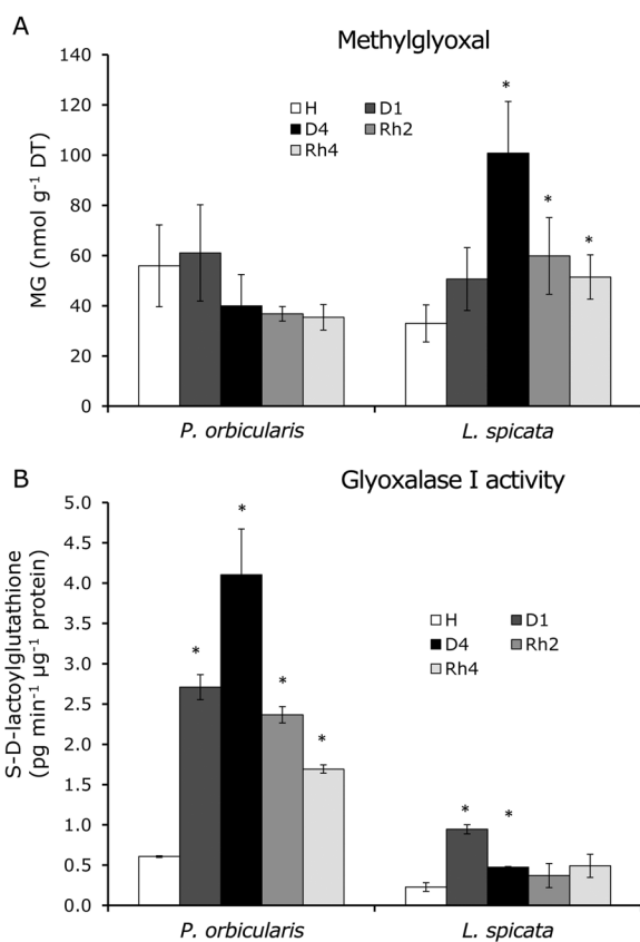
Figure 3. MG concentration (expressed in \text{nmol g}^{-1} DT) (A) and specific activity of GLO1 (expressed as S-D-lactoylglutathione \text{pg min}^{-1} \mu\text{g}^{-1} protein) (B) in P. orbicularis and L. spicata during a desiccation (D)-rehydration (Rh) cycle. The asterisk above the histogram indicates significant differences with hydration at P < 0.05 . DT, dry tissue. Values are mean \pm SD of 5 replicates / Concentración de MG (expresada en \text{nmol g}^{-1} DT) (A) y la actividad específica de GLO 1 (expresada como proteína S-D-lactoilglutathione \text{pg min}^{-1} \mu\text{g}^{-1} ) (B) en P. orbicularis y L. spicata durante un ciclo de desecación (D)-rehidratación (Rh). El asterisco arriba del histograma indica diferencias significativas con hidratación P < 0,05 . DT, tejido seco. Los valores son la media \pm DS de 5 réplicas
