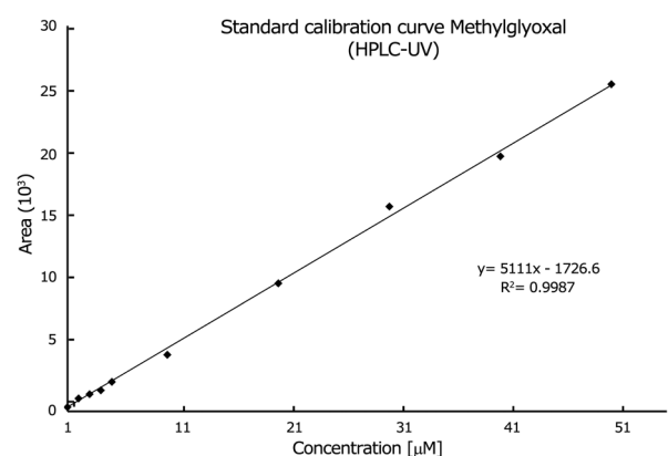
Figure 2. Absolute standard calibration curve obtained for determination of 2-methylquinoxaline, derivatized MG, by HPLC/UV at 334 nm. Values are mean \pm SD of 5 replicates / Curva de calibración estándar absoluta obtenida para la determinación del derivado de 2-metilquinoxalina de MG por HPLC/UV a 334 nm. Los valores son la media \pm DS de 5 réplicas
