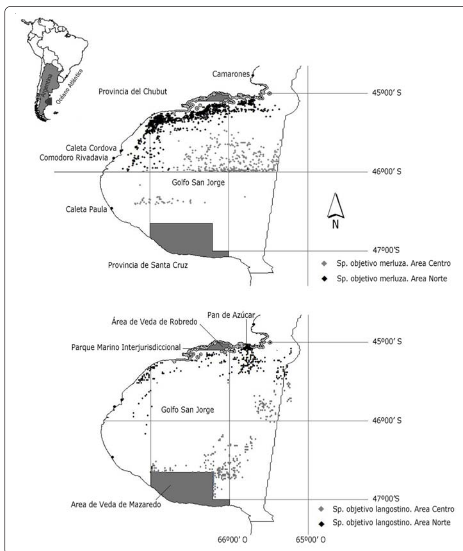
Figura 1. Lances analizados y caracterizados por especie objetivo y área de pesca. Flota fresca de altura, Programa de Observadores a Bordo de la Provincia del Chubut, período 2003-2012 / Hauls analysed and characterized by target species and fishing area. Ice- trawlers fleet, On-board Observer Program of the Chubut Province, during 2003-2012 June period
